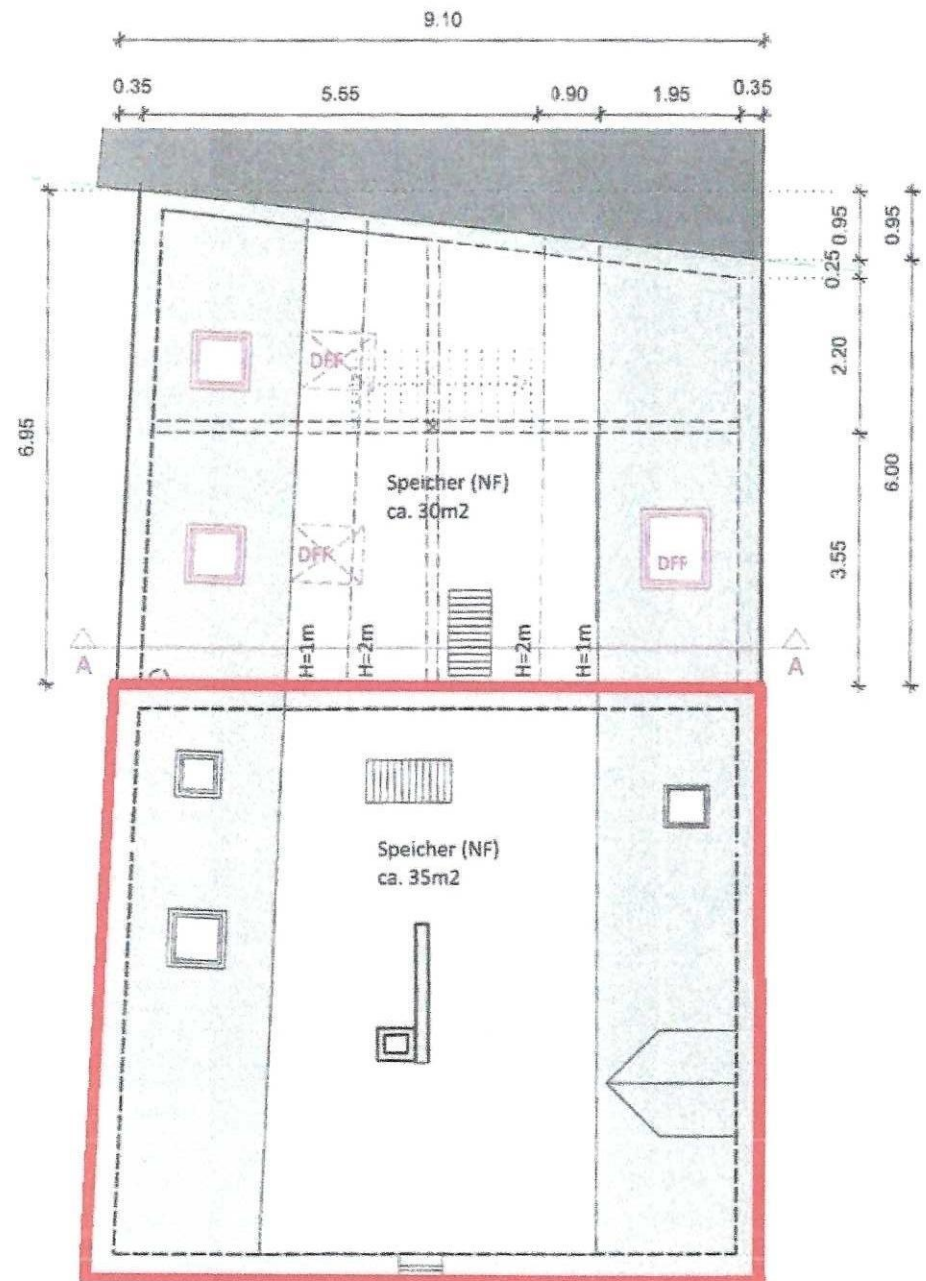
Grundriss DG
