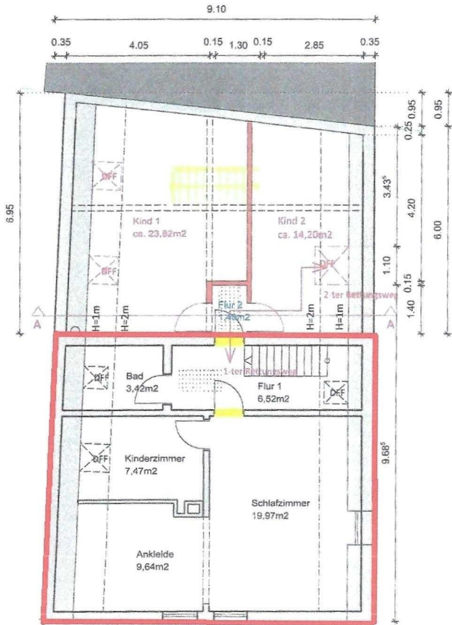
Grundriss 2.OG
